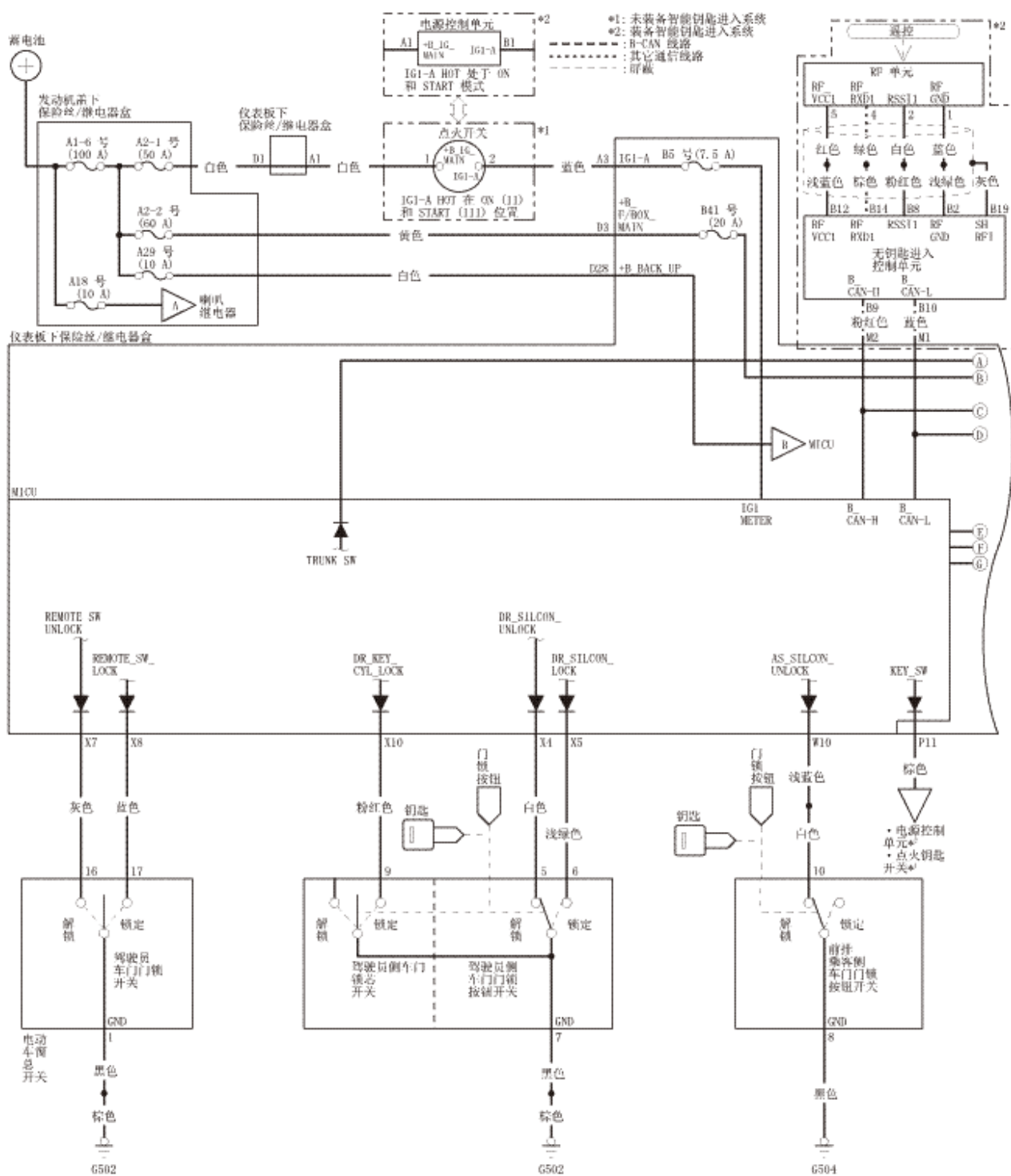
智能钥匙/电动车门门锁/防盗报警系统电路图
